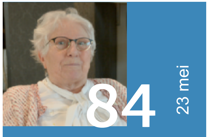
Vivaldi
